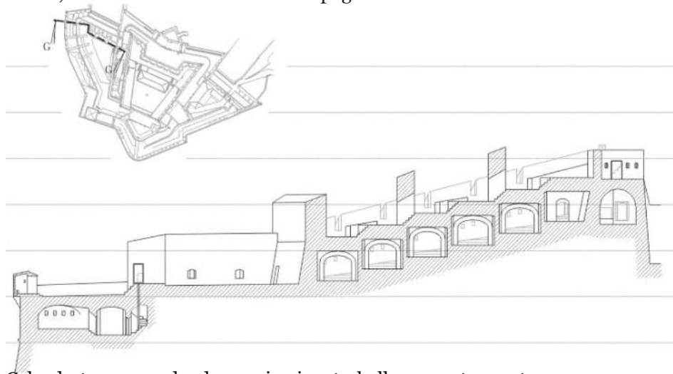
Sección e planta correspondentes ao traballo de levantamento topográfico do castelo de S. Felipe, realizado polos alumnos do módulo profesional de Traballo de Campo e Gabinete baixo a dirección de Alfonso Fuentes
